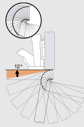
CLIP top BLUMOTION 110° Thin Door Hinge
