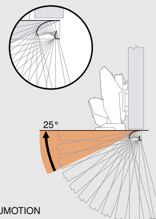
CLIP top BLUMOTION 110° Thin Door Hinge
